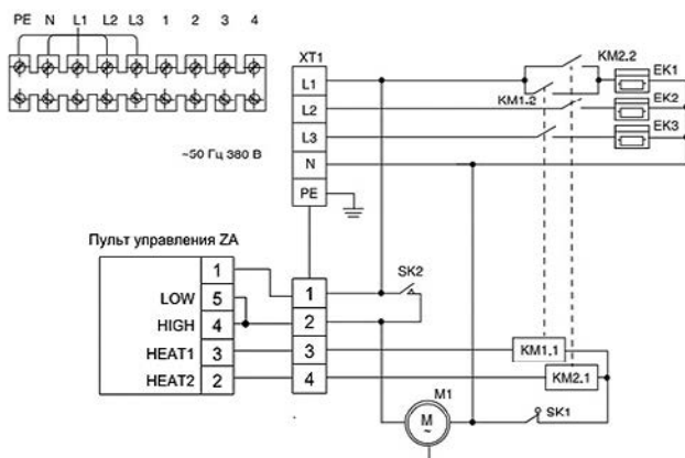
РИС. 5 Схема электрическая ZVV-1E6T, ZVV-1.5E9T, ZVV-2E12T
