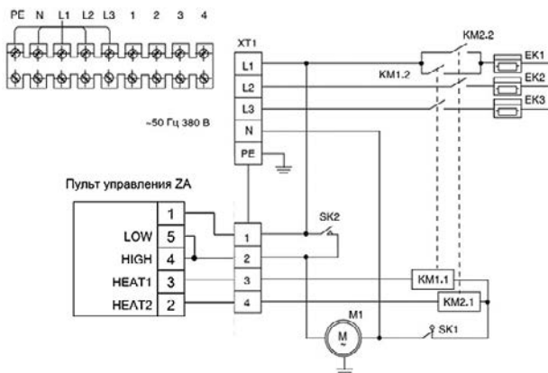
РИС. 6 Схема электрическая ZVV-2E18T, ZVV-2E24T
