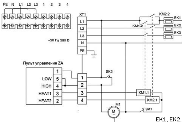
РИС. 5 Схема электрическая ZVV-6T, ZVV-9T, ZVV-12T
