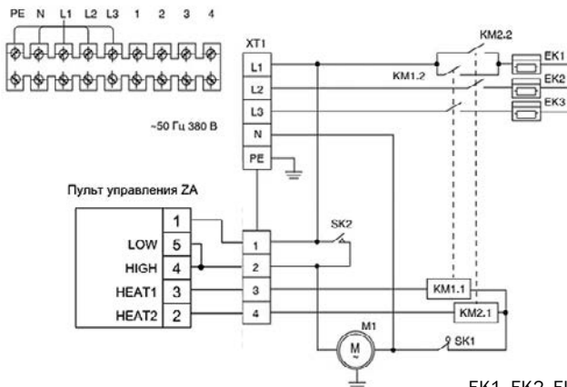
РИС. 6 Схема электрическая ZVV-18T, ZVV-24T
